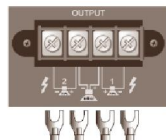
Винтовой клеммный зажим
